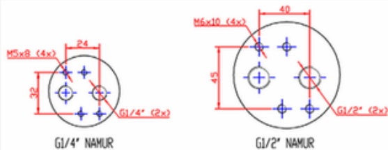
DETALHE A
